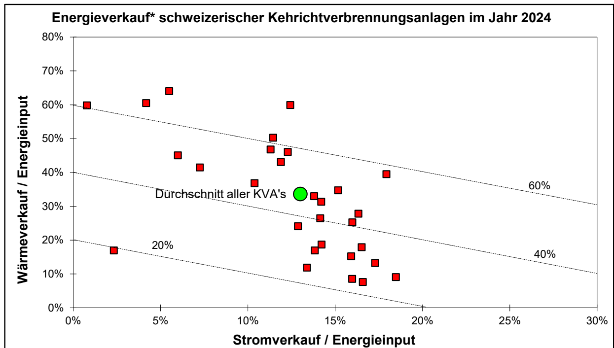
Bild 7.1d Energieverkaufs-Benchmark schweizerischer KVA (Jahr 2024)
