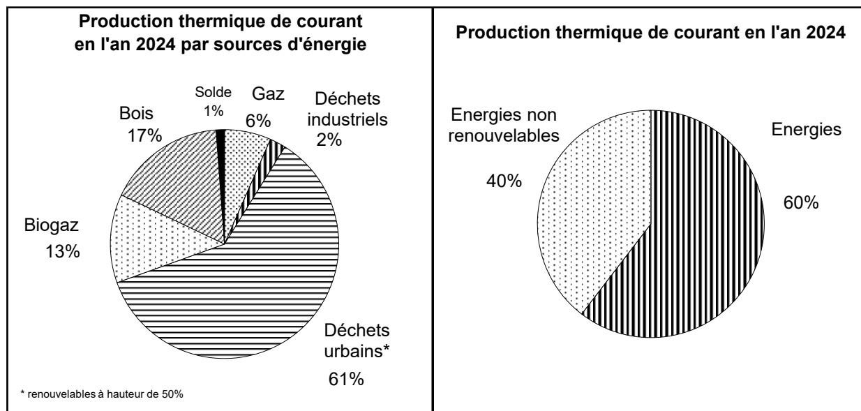
Figure 1.4 Apport des différentes sources d'énergie à la production thermique de courant en 2024
