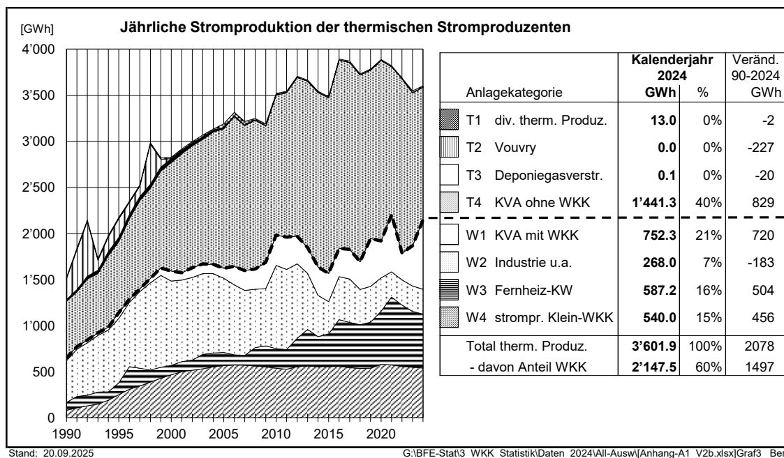
Bild 3.2a Thermische Stromproduktion der Jahre 1990 bis 2024
