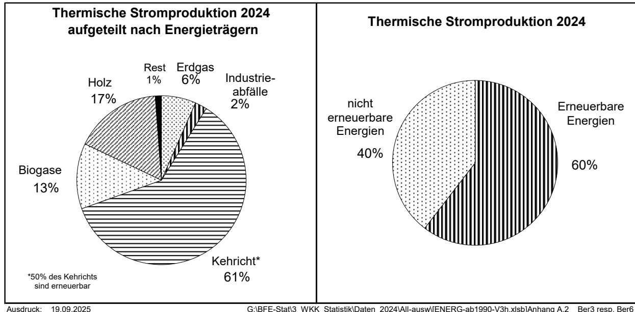
Bild 1.4 Aufteilung der thermischen Stromproduktion des Jahres 2024 nach Energieträgern
