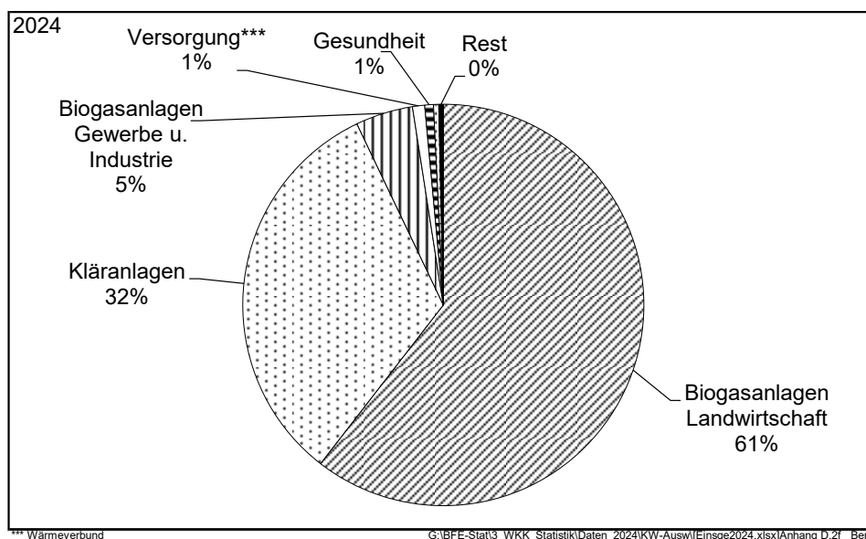
Bild 6.2d Neuinstallierte Klein-WKK-Leistung nach Einsatzgebieten (Jahr 2024)
