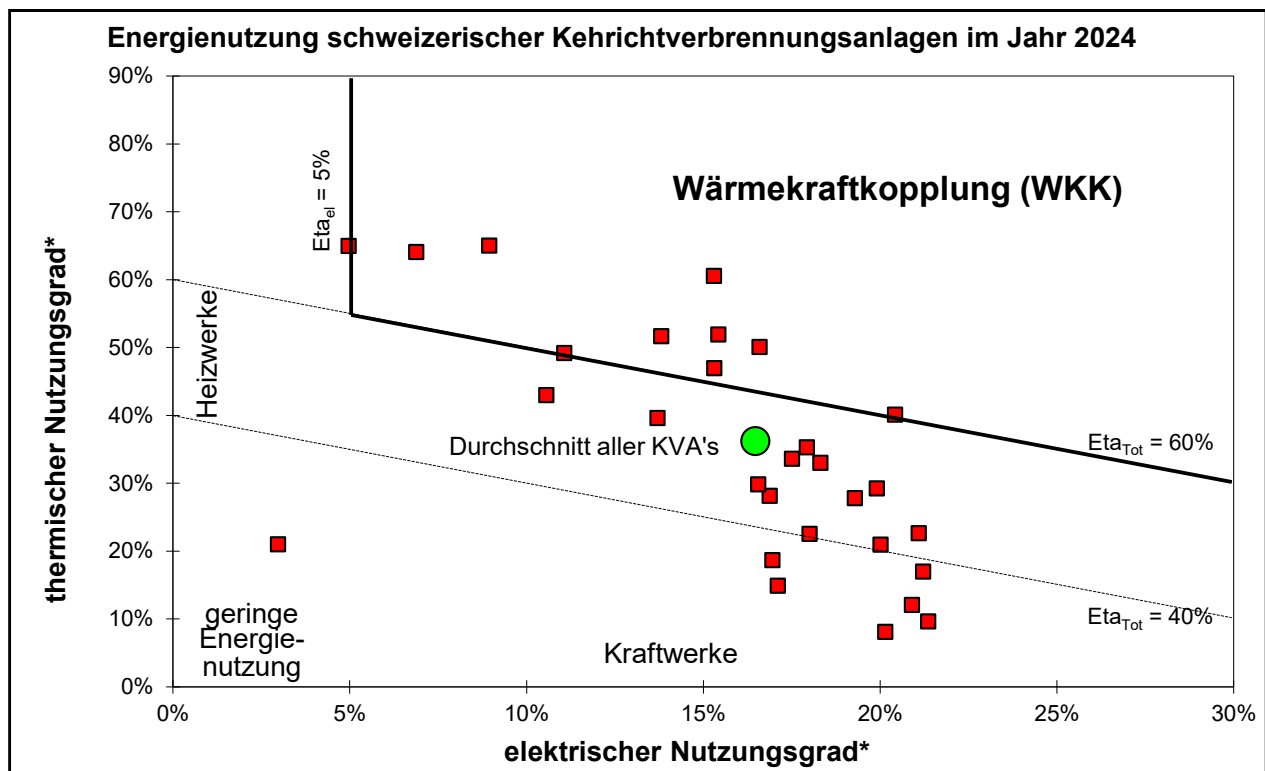
Bild 2.3 Jahresnutzungsgrade der schweizerischen Kehrichtverbrennungsanlagen im Jahr 2024
