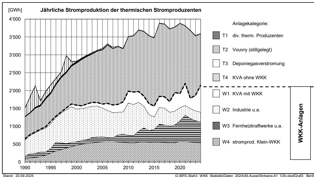
Bild 1.3 Entwicklung der thermischen Stromproduktion
