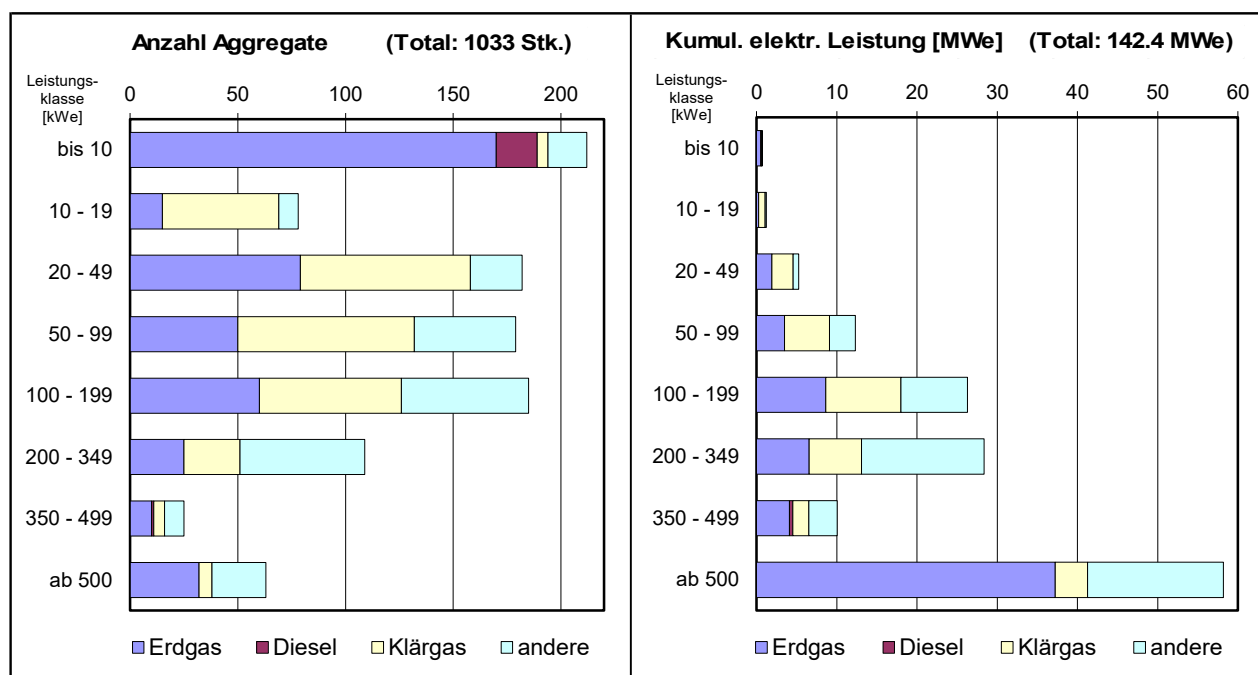
Bild 6.1f Ende 2024 in Betrieb stehende Klein-WKK-Aggregate, geordnet nach Leistungsklassen und nach Energieträgern
